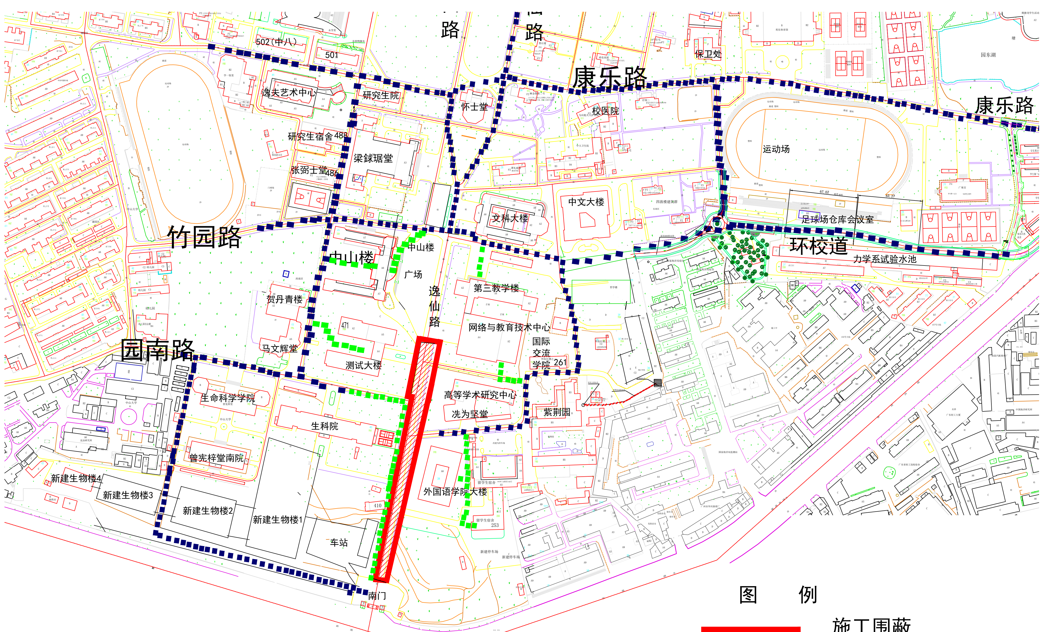
南校园逸仙路、岭南路西段（含博物馆周边）道路维修工程 ——逸仙路南段第三施工段交通围蔽方案
